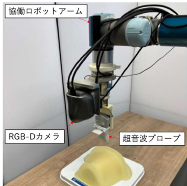
超音波検査支援ロボット
