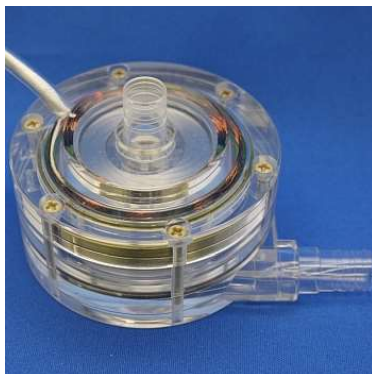
中長期の心肺補助を目指した動圧浮上遠心血液ポンプ
